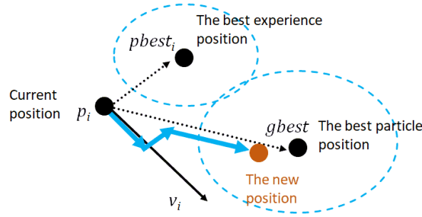
Gambar 2.8: Ilustrasi perpindahan satu partikel berdasarkan velocity baru yang dipengaruhi oleh personal best dan global best .
